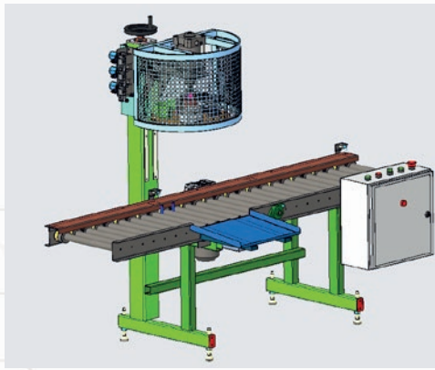
Автомат проверки герметичности тары Pails leak testing machine
