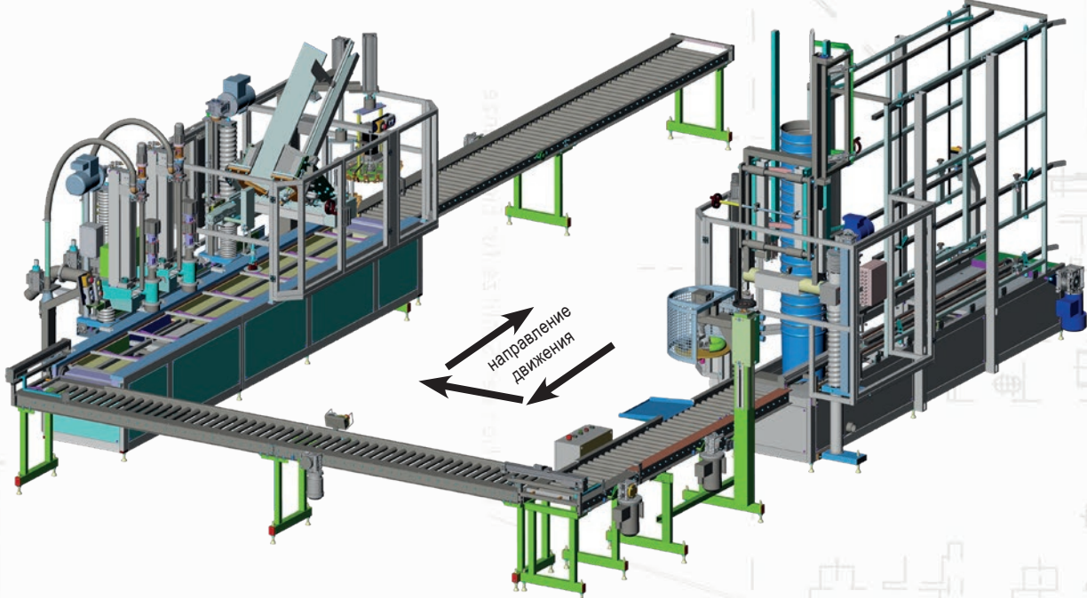
Автомат проверки герметичности тары Pails leak testing machine
