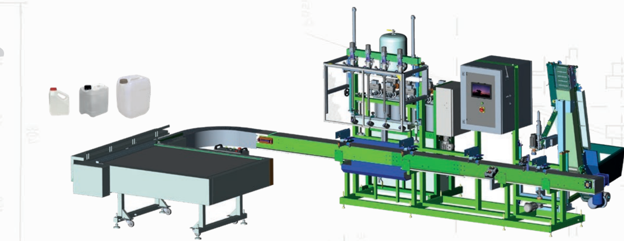
Filling system LR.3-04 Линия розлива и укупорки ЛР.3-04
