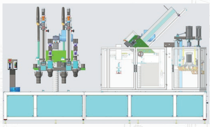
Автомат дозирования с двумя комплектами клапанов для дозирования жидких пенящихся и вязких продуктов Automatic filling machine with two types of dosing nozzles for dosing foam liquids and viscous products
